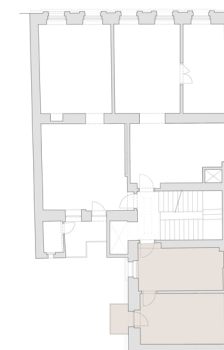
půdorys podlaží
